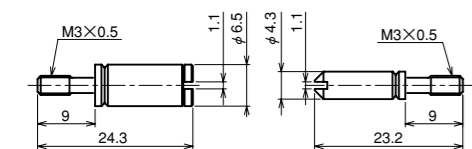
■1 インサート又は、1 モジュールフレームのガイドピン/ガイドブッシュ取付組合せ図
