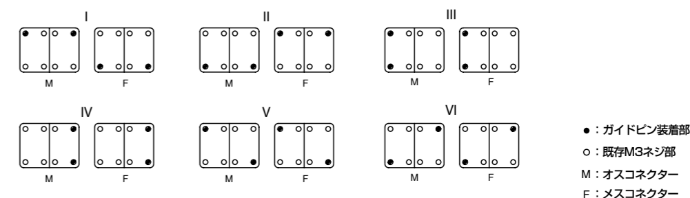
■2 インサート又は、2 モジュールフレームのガイドピン取付組合せ図
