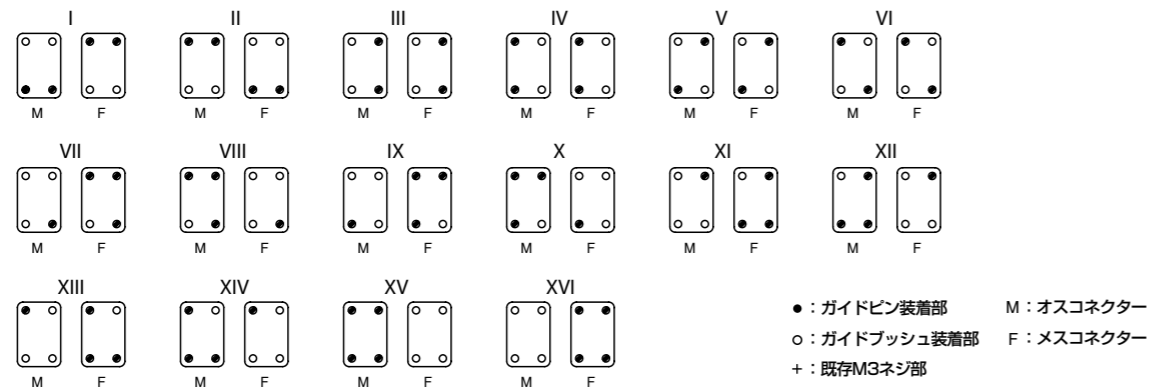
■2 インサート又は、2 モジュールフレームのガイドピン/ガイドブッシュ取付組合せ図
