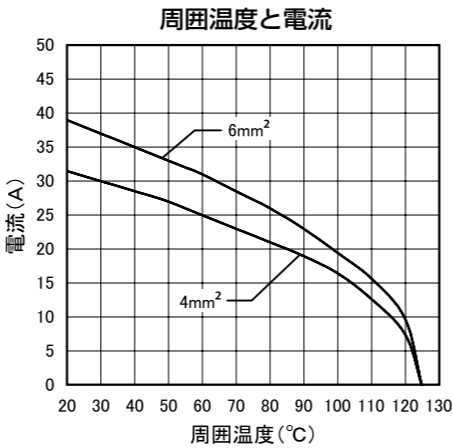
YSF※24Bに6モジュール取付け時
