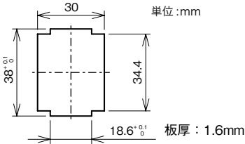
取付け1個穴
