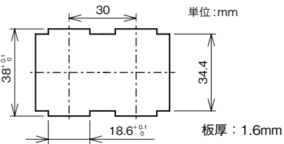
取付け2個穴
