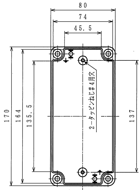
A-A (BOX内部)
