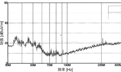
〈 电缆 〉
