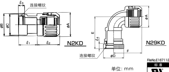
单位: mm
