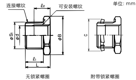
无锁紧螺母
